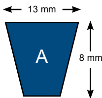
PERFIL A 13 x 8 mm/BLADE
