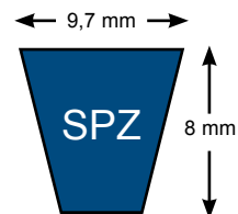
PERFIL SPZ 9,7 x 8 mm/BLADE
